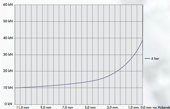
Kraftverlauf KP3.1N
