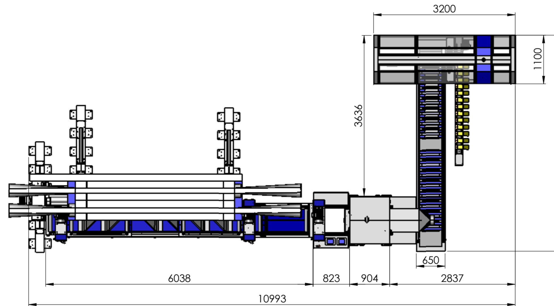
HEFTEC CPM530 Präzisionsstanzmaschine
